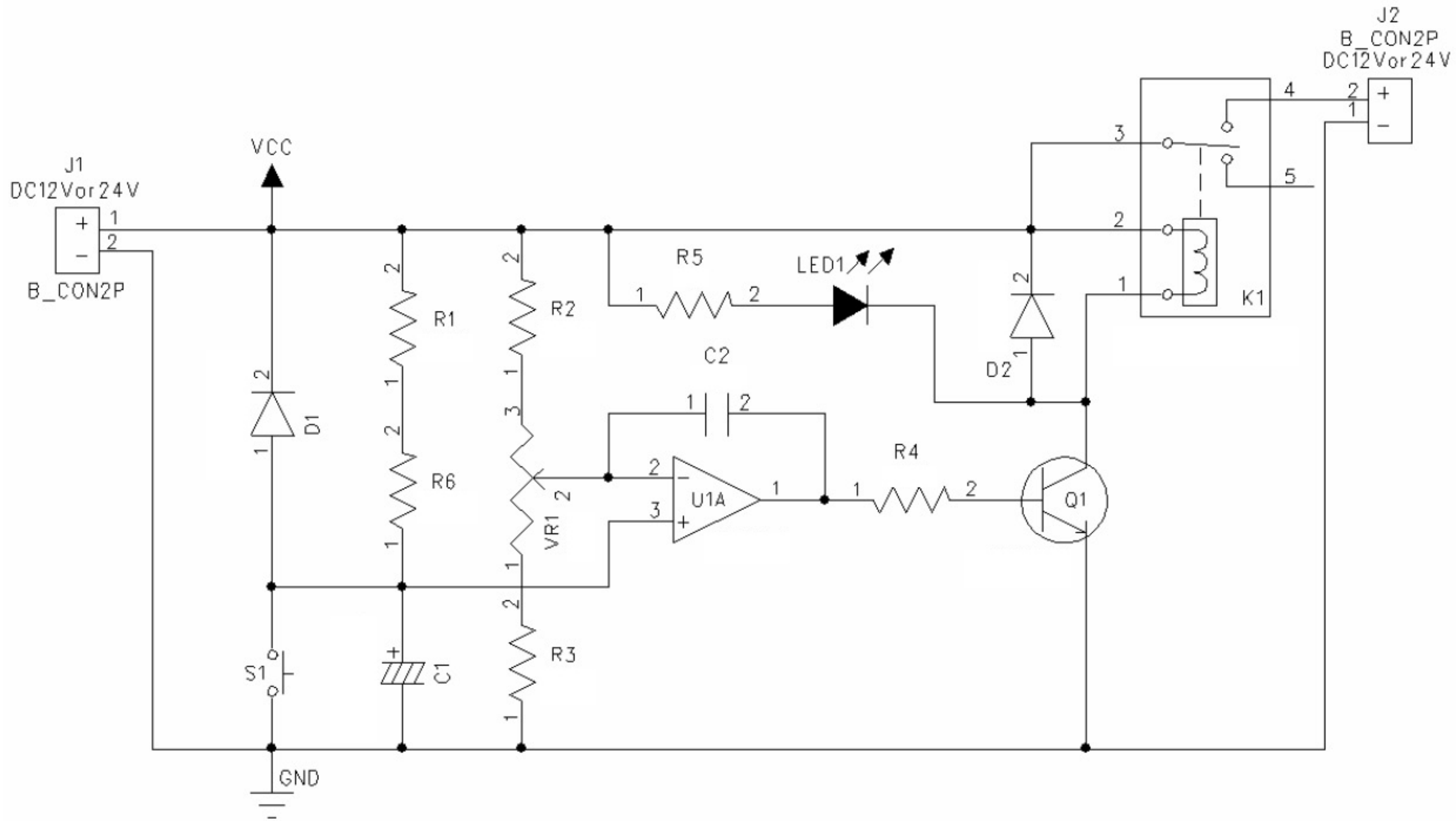
FK-5103/5108 회로도
